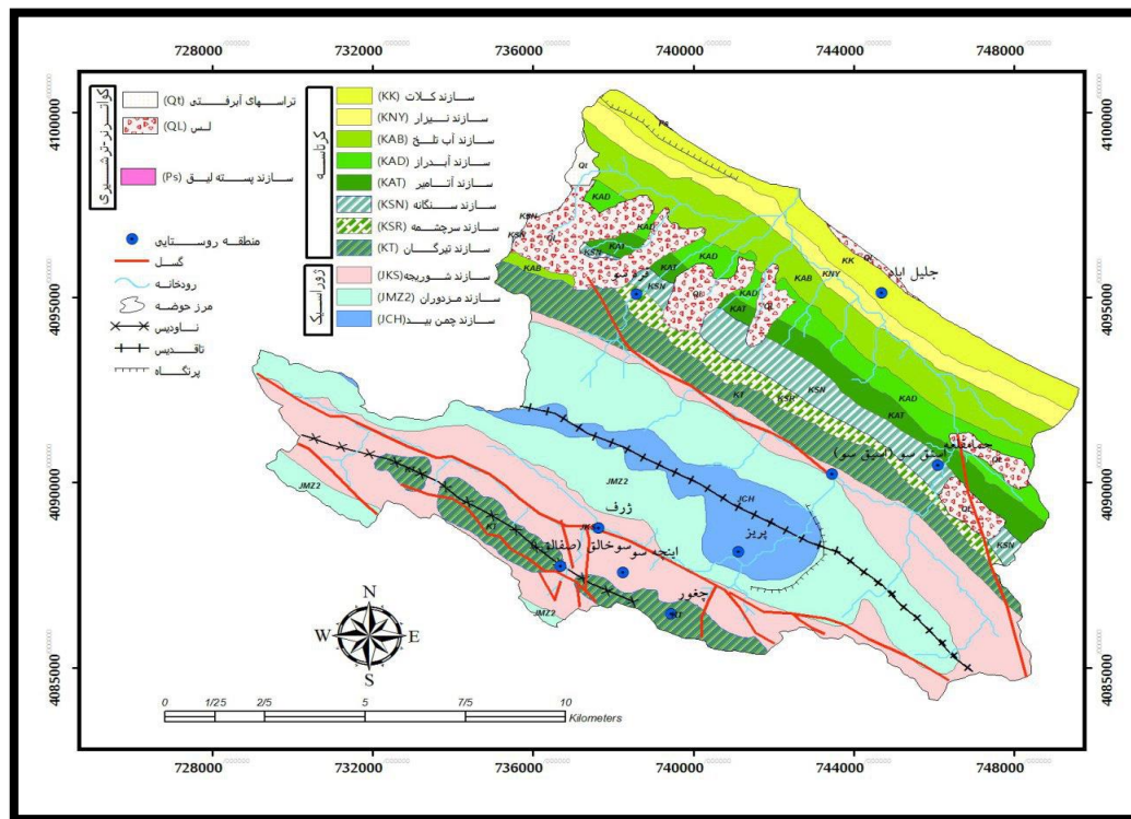
شکل ۲: نقشه زمین شناسی حوزه کوهستانی کلات (مأخذ: نقشه زمین شناسی ۱:۱۰۰۰۰۰ کلات سازمان زمین شناسی و اکتشافات معدنی کشور)
