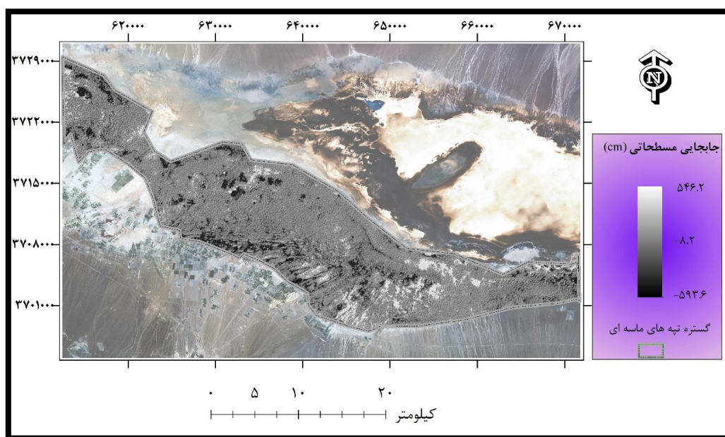
شکل ۵: نقشه جابجایی مسطحی تپه‌های ماسه‌ای حاصل از تداخل سنجی راداری تصاویر Sentinel 1
