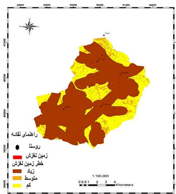
شکل ۴: نقشه پهنه‌بندی خطر در مدل آماری نسبت فراوانی
