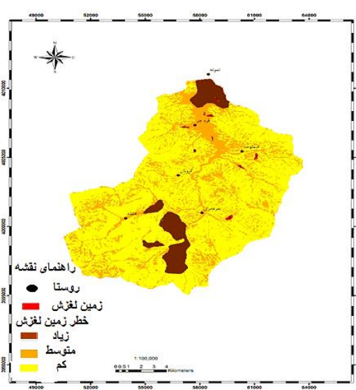
شکل ۵: نقشه پهنه‌بندی خطر در مدل تراکم سطح
