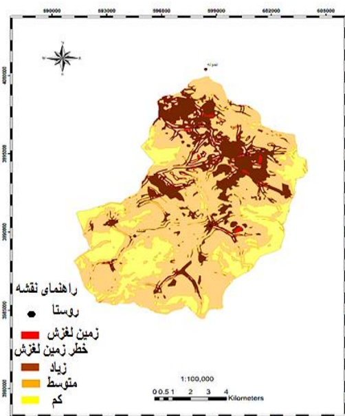
شکل ۳: نقشه پهنه‌بندی خطر در مدل LNRF
