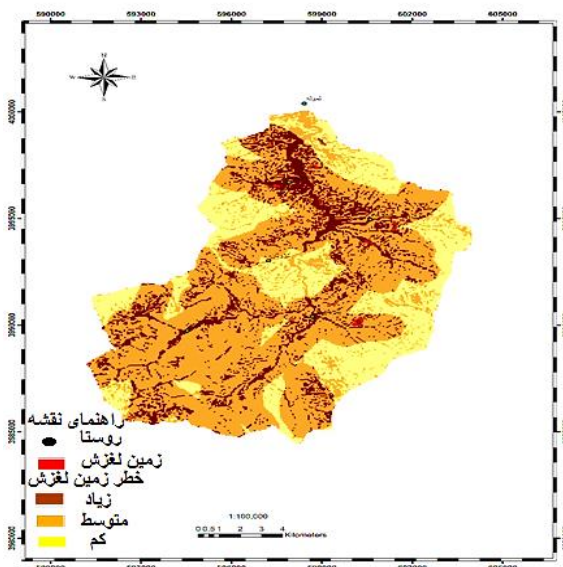
شکل ۶: نقشه پهنه‌بندی خطر در مدل ارزش اطلاعات
