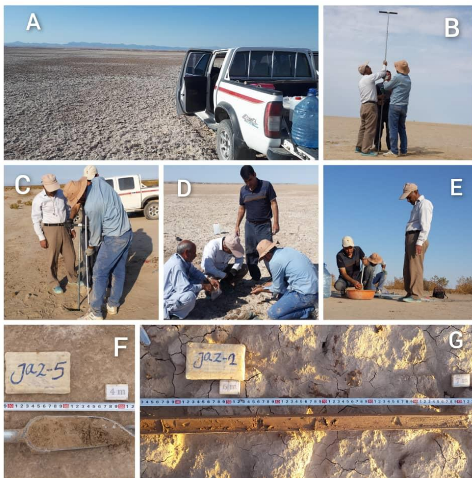
شکل ۴. A: نمایی از پلاایای جازموریان، B: نحوه قرار گیری افراد و انجام مغزه گیری، C: اندازه گیره عمق و ضخامت برداشت مغزه، D: توصیف رسوبات حفاری شده، E: انجام شستشو بعد از هر بار مغزه گیری جهت جلوگیری از الودگی های احتمالی با رسوبات بالایی و زیرین در توالی رسوبی، F: نمونه ای از مغزه خارج شده از چاه (Soil auger)، G: نمونه ای از مغزه برداشت شده (Gouge auge)
