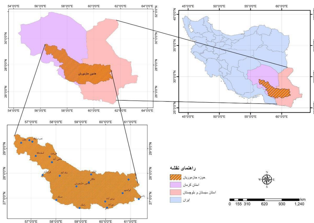
شکل ۱: حوضه آبریز پلایای جازموریان و موقعیت آن در تقسیم‌بندی استان‌های کشور (ترسیم نگارندگان)
