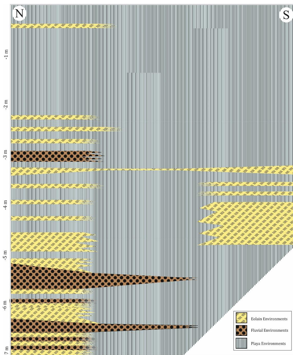
شکل ۱۰: انطباق تقریبی شمالی - جنوبی محیط‌های رسوبی در مغزه‌های برداشت شده در پلاهای جازموریان
