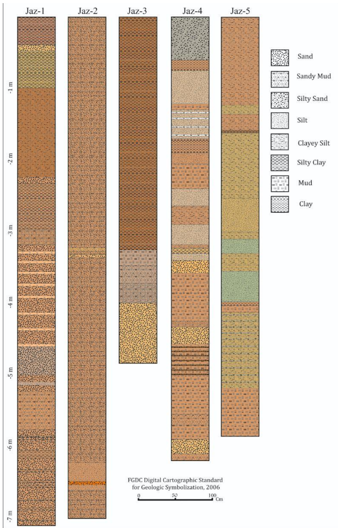
شکل ۶: ستون چینه‌ای مغزه‌های برداشت‌شده از پلایای جازموربان
