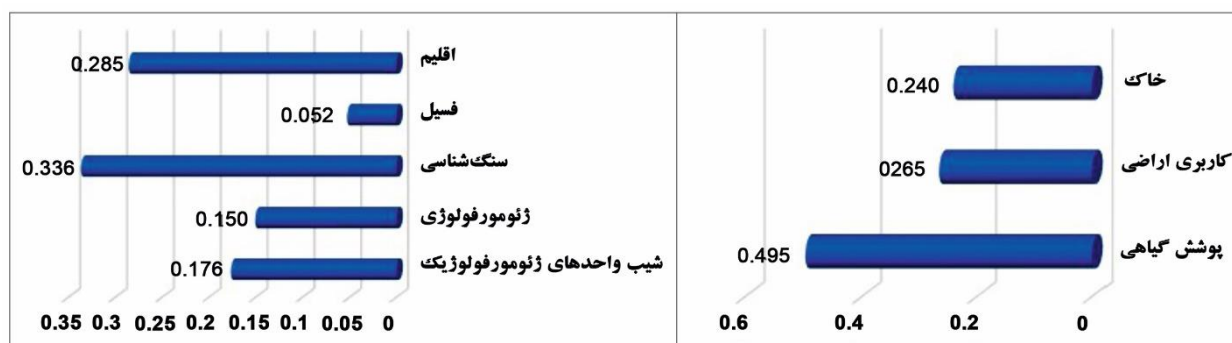
شکل ۶: وزن نسبی زیرمعیارهای تنوع زمینی پهنه کبه‌داغ شرقی در استان خراسان رضوی
