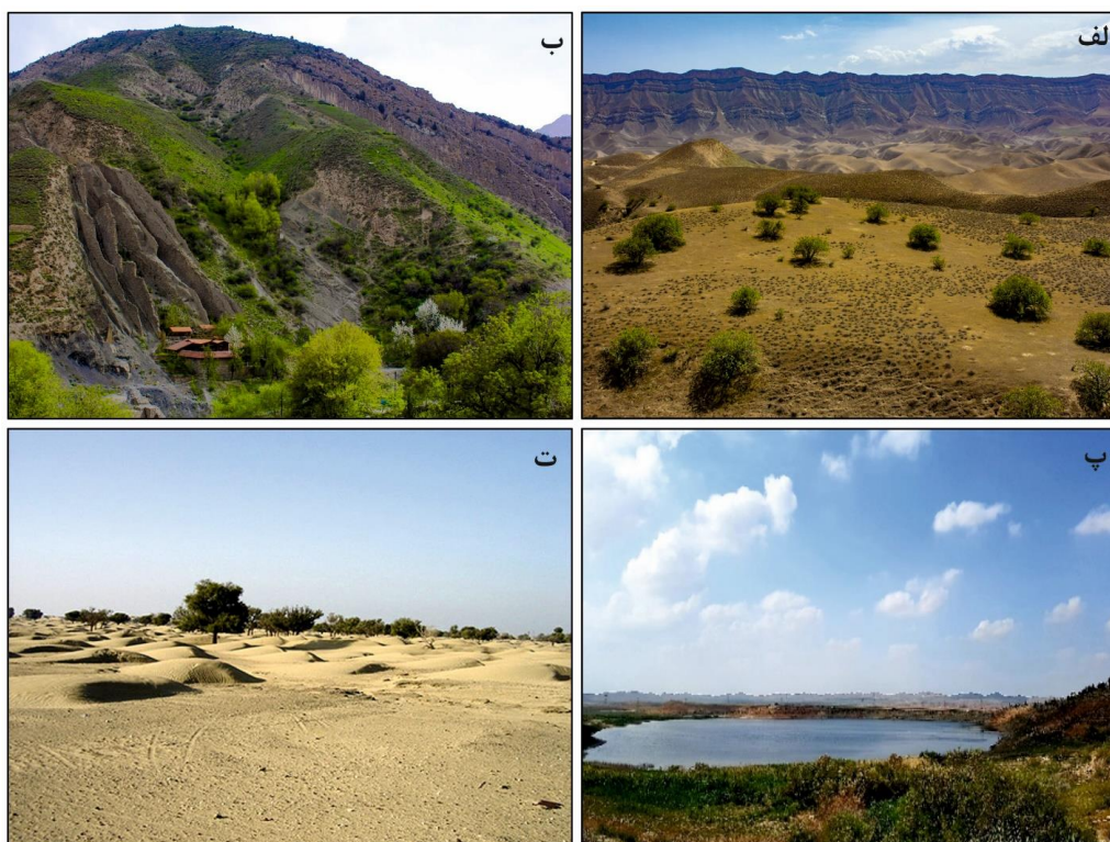
شکل ۲: تصاویری از چشم‌اندازهای طبیعی پهنه کپه‌داغ شرقی در استان خراسان رضوی؛ (الف) جنگل درخت‌های یسته موسوم به جنگل خواجه در پیرامون جاده مشهد - سرخس؛ (ب) فرسایش تفریقی در سنگ آهک‌ها و تیل‌های سازند سرچشمه در مسیر آبشار قره‌سو - کلات نادری؛ (پ) دریاچه بزنگان در خاور جاده مشهد - سرخس، شمال روستای بزنگان؛ (ت) چشم‌انداز حاصل از جابجایی ماسه‌ها در بیابان‌های اطراف شهر سرخس
