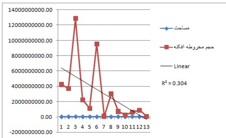
شکل ۵. رابطه‌ی خطی بین مساحت حوضه‌ی بالادست مخروطها (BA) و حجم مخروط افکنه‌ها (V) حوضه‌ی اردستان
