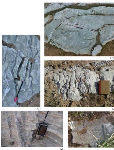
شکل ۲- (الف) و (ب)، ریل کارن‌ها در رخنمون‌های سطحی گچ (ج)، حرکت موجی رانل‌های گچی، (د) و (ه)، وال کارن‌ها روی دیواره عمودی یک فروچاله ریزشی در لایه‌های گچی سازند گچساران، منطقه آسماری، جنوب شرق مسجد سلیمان، استان خوزستان.
