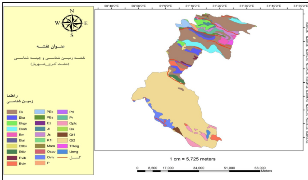
شکل ۲: وضعیت زمین‌شناسی - چینه‌شناسی حوضه و دشت کرج - شهریار
