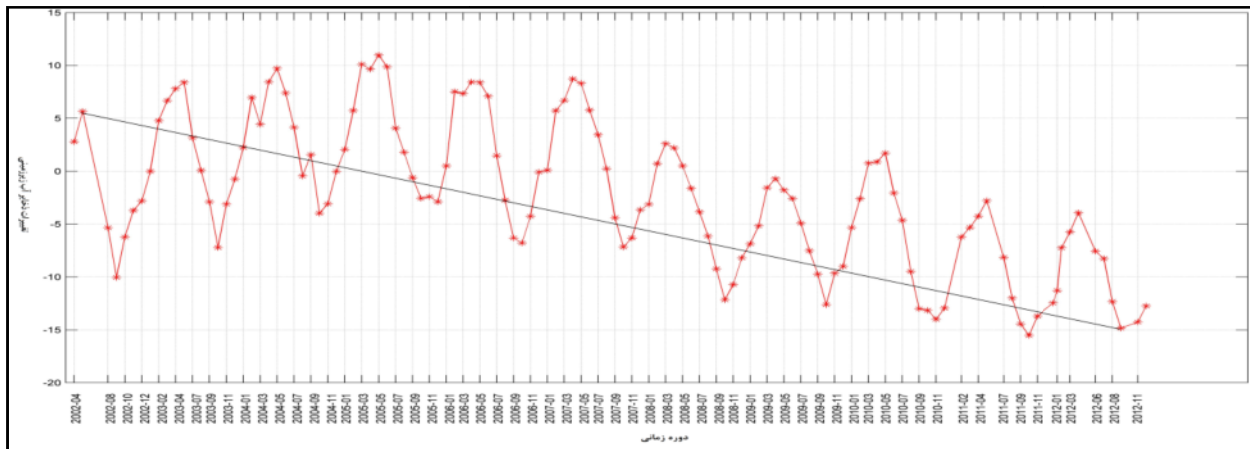
شکل ۳: روند میزان افت آب طی سال‌های ۲۰۰۲ تا ۲۰۱۲
