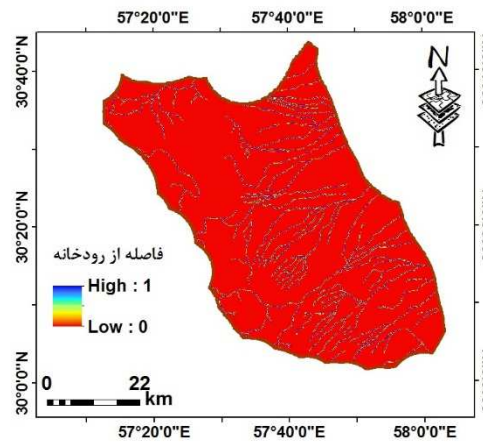
رودخانه
