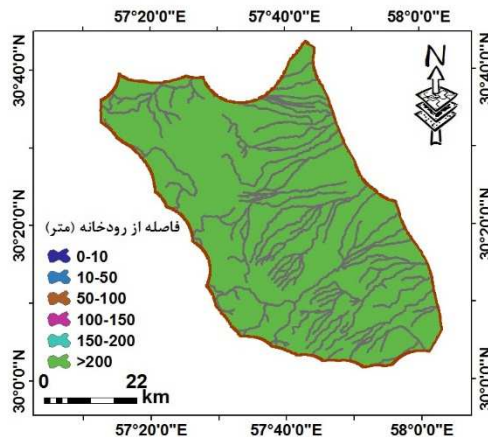
رودخانه
