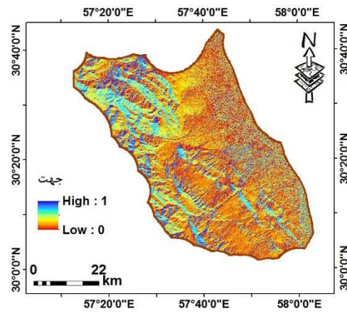
جهت شیب
