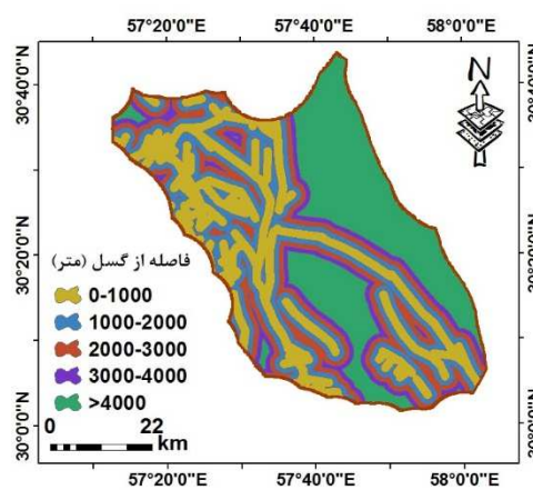
گسل
