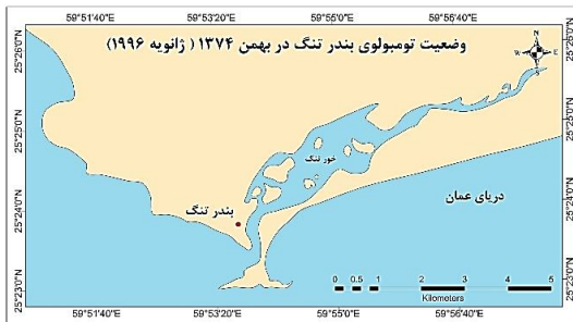
شکل ۲۲: وضعیت ژئومورفولوژیکی تومبولوی بندر تنگ در بهمن ۱۳۷۳ شکل ۲۳: وضعیت ژئومورفولوژیکی تومبولوی بندر تنگ در بهمن ۱۳۷۴
