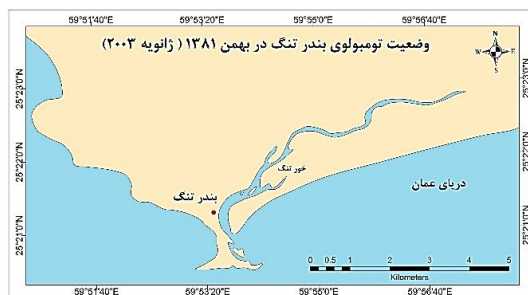
شکل ۳۰- وضعیت ژئومورفولوژیکی تومبولوی بندر تنگ در بهمن ۱۳۸۱ (ژانویه ۲۰۰۳) وضعیت تومبولوی بندر تنگ در اردیبهشت ۱۳۸۲ (آوریل ۲۰۰۴)
