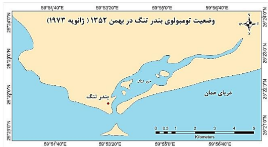
شکل ۵: وضعیت ژئومورفولوژیکی تومبولوی بندر تنگ در بهمن ۱۳۵۲
