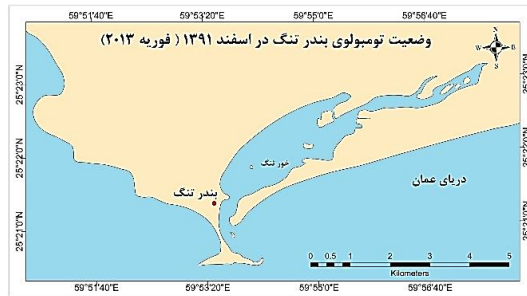
شکل ۴۰- وضعیت ژئومورفولوژیکی تومبولوی بندر تنگ در اسفند ۱۳۹۱
