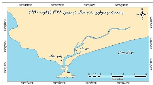
شکل ۱۷: وضعیت ژئومورفولوژیکی تومبولوی بندر تنگ در بهمن ۱۳۶۸
