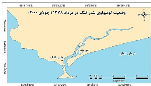
شکل ۲۶: وضعیت ژئومورفولوژیکی تومبولوی بندر تنگ در بهمن ۱۳۷۷ شکل ۲۷: وضعیت ژئومورفولوژیکی تومبولوی بندر تنگ در مرداد ۱۳۷۸
