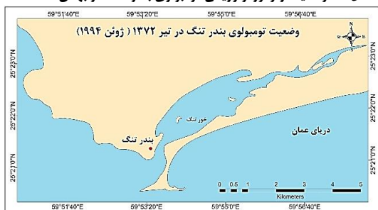
شکل ۲۱: وضعیت ژئومورفولوژیکی تومبولوی بندر تنگ در تیر ۱۳۷۲
