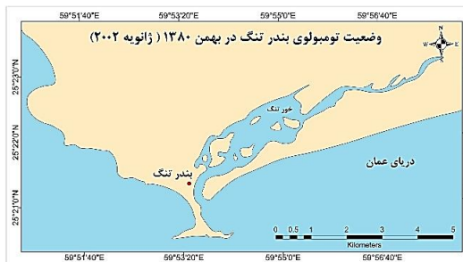
شکل ۲۸: وضعیت ژئومورفولوژیکی تومبولوی بندر تنگ در تیر ۱۳۷۹ شکل ۲۹: وضعیت ژئومورفولوژیکی تومبولوی بندر تنگ در بهمن ۱۳۸۰
