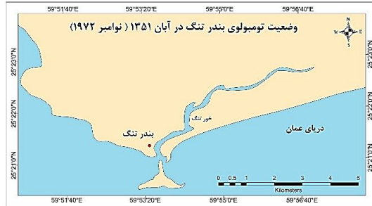
شکل ۴: وضعیت ژئومورفولوژیکی تومبولوی بندر تنگ در آبان ۱۳۵۱ (نوامبر ۱۹۷۲)
