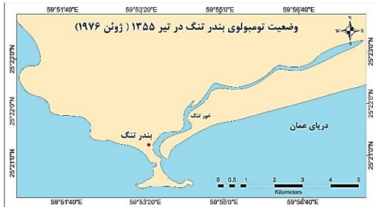
شکل ۷: وضعیت ژئومورفولوژیکی تومبولوی بندر تنگ در تیر ۱۳۵۵
