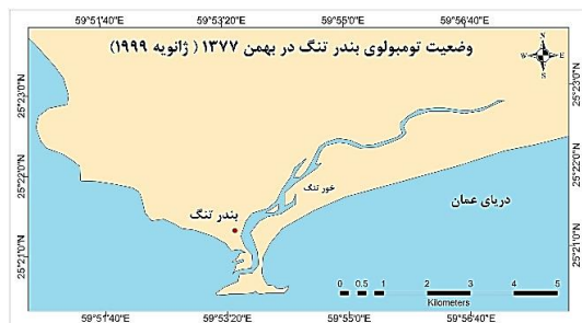
شکل ۲۶: وضعیت ژئومورفولوژیکی تومبولوی بندر تنگ در بهمن ۱۳۷۷ شکل ۲۷: وضعیت ژئومورفولوژیکی تومبولوی بندر تنگ در مرداد ۱۳۷۸
