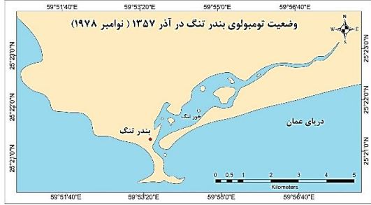
شکل ۹: وضعیت ژئومورفولوژیکی تومبولوی بندر تنگ در آذر ۱۳۵۷
