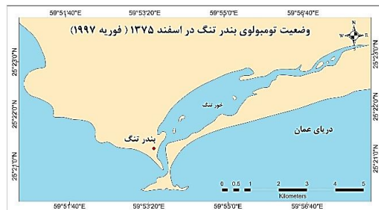
شکل ۲۴: وضعیت ژئومورفولوژیکی تومبولوی بندر تنگ در اسفند ۱۳۷۵ شکل ۲۵: وضعیت ژئومورفولوژیکی تومبولوی بندر تنگ در تیر ۱۳۷۶
