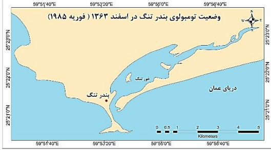
شکل ۱۲: وضعیت ژئومورفولوژیکی تومبولوی بندر تنگ در اسفند ۱۳۶۳
