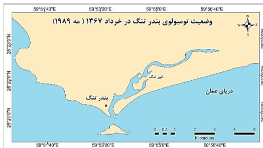
شکل ۱۶: وضعیت ژئومورفولوژیکی تومبولوی بندر تنگ در خرداد ۱۳۶۷
