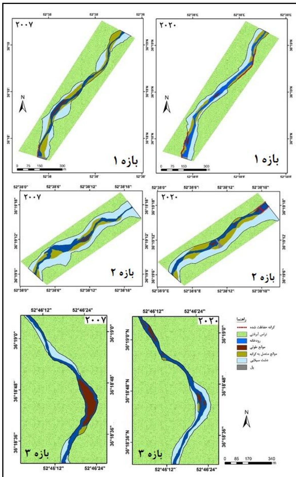
شکل ۲: نقشه‌های ژئومورفولوژی رودخانه بابلرود در بازه‌های مورد مطالعه در دو سال ۲۰۰۷ و ۲۰۲۰
