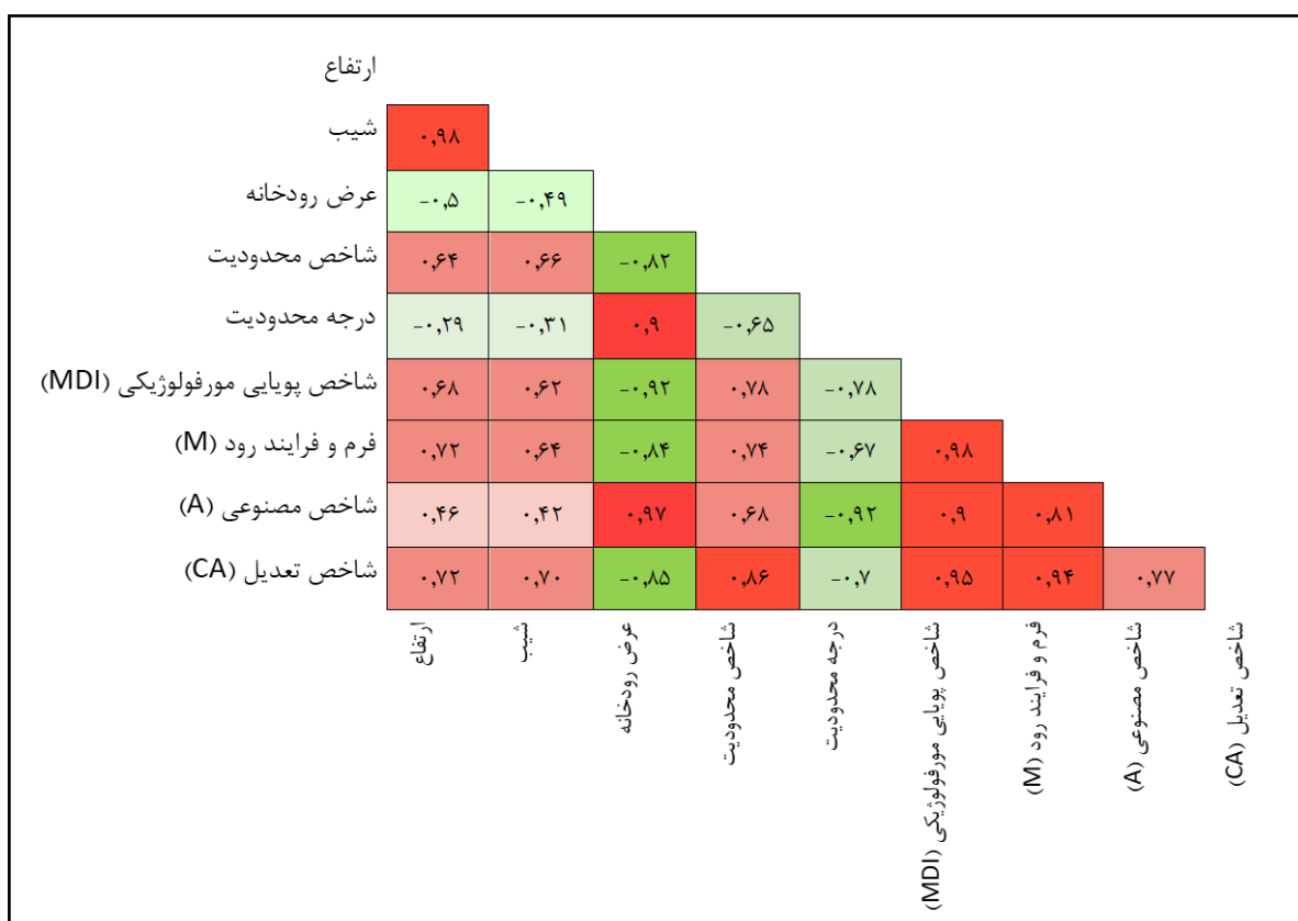
شکل ۶: ضریب همبستگی پیرسون بین متغیرهای مختلف و شاخص‌های پویایی مورفولوژیکی رود در رودخانه بابلرود
