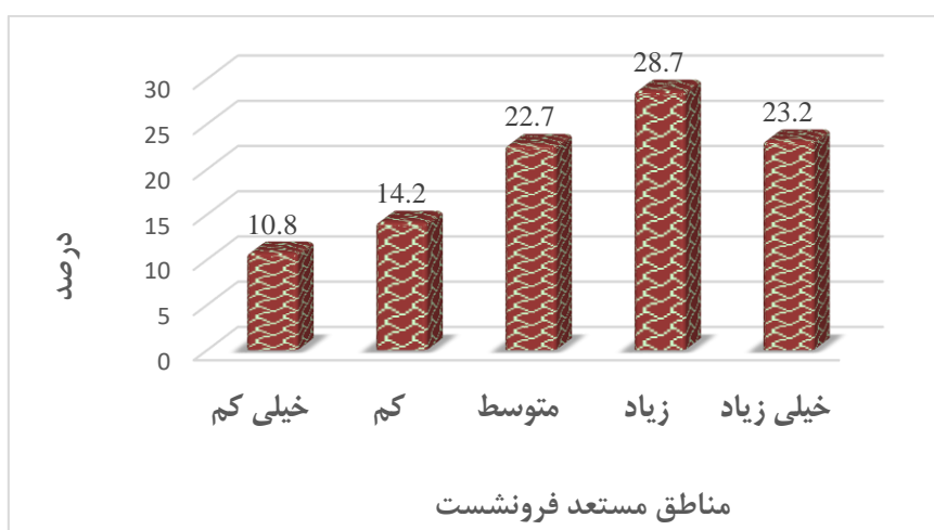
شکل ۱۳: نمودار درصد مناطق مستعد فرونشست محدوده مطالعاتی با روش AHP-FUZZY
