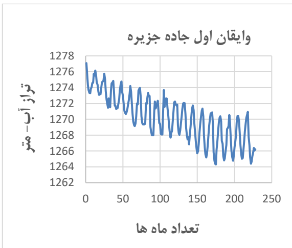
شکل ۹: نمودارهای سری زمانی چاه‌های مشاهداتی دارای افت آب و فرونشست در محدوده مطالعاتی
