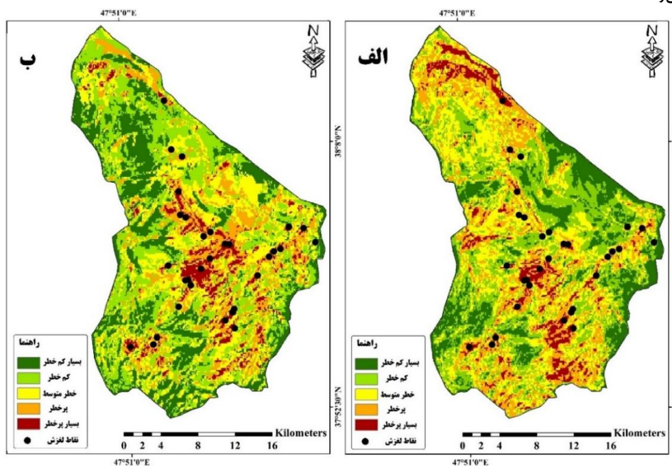
شکل ۸: نقشه پهنه‌بندی خطر زمین‌لغزش حوضه بالادست سد یامچی؛ (الف) خروجی حاصل از روش MARCOS (ب) خروجی حاصل از روش CODAS
