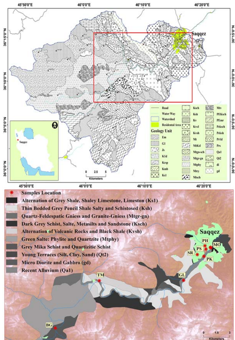
شکل ۱. موقعیت جغرافیایی و نقشه زمین شناسی حوضه آبخیز رودخانه سقز، بازه مورد بررسی و نمونه‌های برداشت شده (BG، TM و GL نمونه‌های رسوبات جدید دشت سیلابی؛ SR، PK، PS، PH و MO نمونه‌های رسوبات قدیم دشت سیلابی). در هر کدام از محل‌های اتصال شاخه‌ها به شاخه اصلی دو نمونه رسوب از بخش گراولی و ما سه‌ای رسوبات جدید دشت سیلابی برداشت گردید؛ نمونه‌های رسوبات قدیمی دشت سیلابی هم با توجه به محل رخنمون آن‌ها، در پایین دست حوضه (محدوده شهر سقز و اطراف آن) جمع‌آوری شدند.
