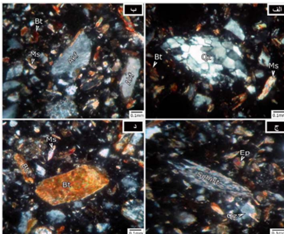
شکل ۵. الف) دانه فلدسپات در مجاورت خردسنگ اسلیتی؛ ب) نمایی از یک خردسنگ شیستی در کنار خردسنگ بلوری کوارتز؛ ج) نمایی از یک خردسنگ آتشفشانی و دانه کوارتز که هر دو گرد شدگی خوبی نشان می‌دهند؛ د) بلور پلاژیوکلاز نیمه‌گرد شده در نزدیکی بلور مسکوویت و خردسنگ شیستی در بین آن‌ها.
