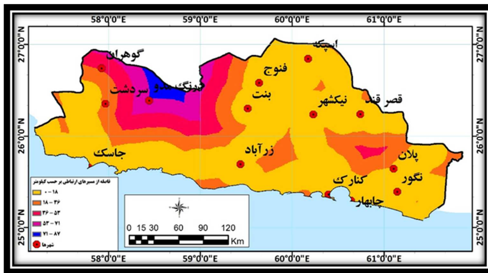
شکل ۱۳: نزدیکی به مسیرهای ارتباطی
