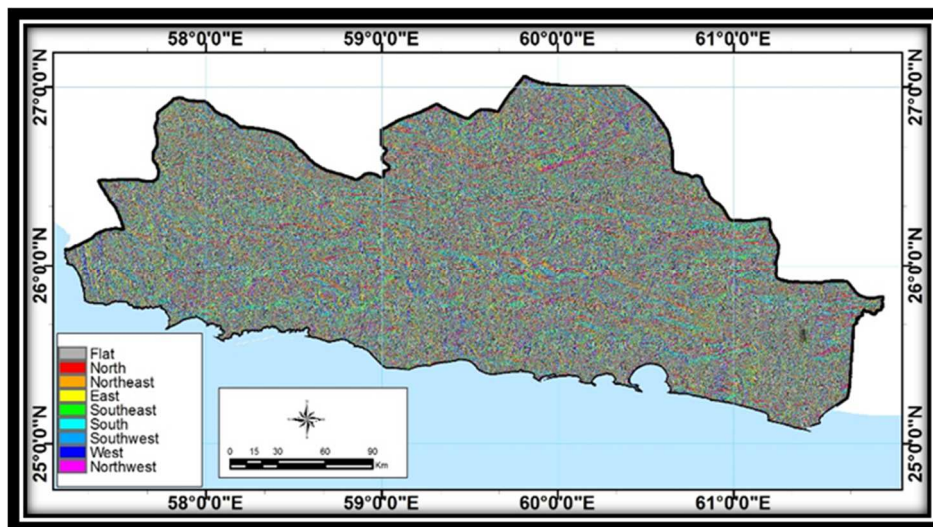
شکل ۸: تقسیم‌بندی منطقه مورد مطالعه براساس جهات شیب
