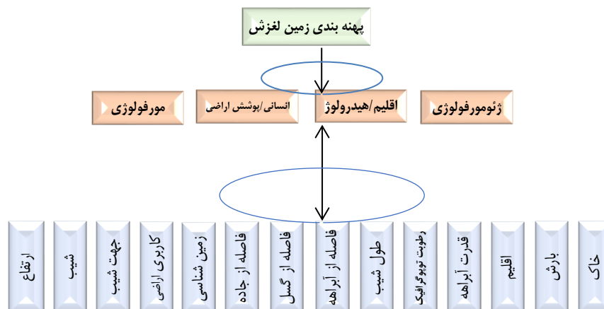
شکل ۳: نمودار معیارها و زیر معیارهای ارزیابی پتانسیل زمین لغزش‌های پهنه لرزه‌ای ارسباران
