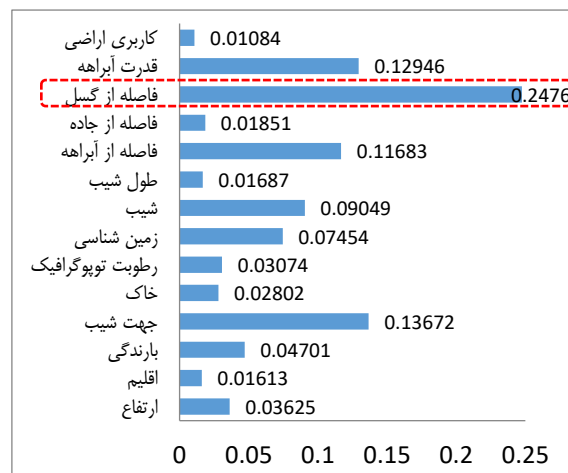
شکل ۱۷: ضرایب استخراج شده از مدل تحلیل شبکه
