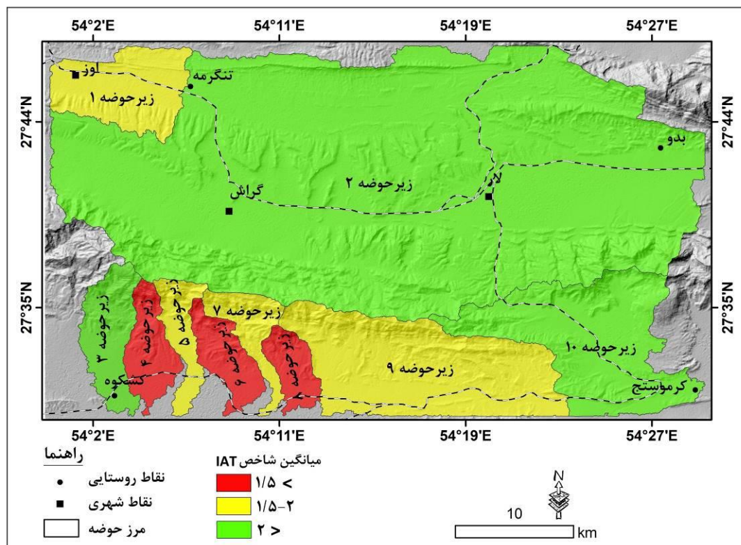
نقشه ۳: نمودار میانگین شاخص IAT در زیرحوضه‌های مورد مطالعه
