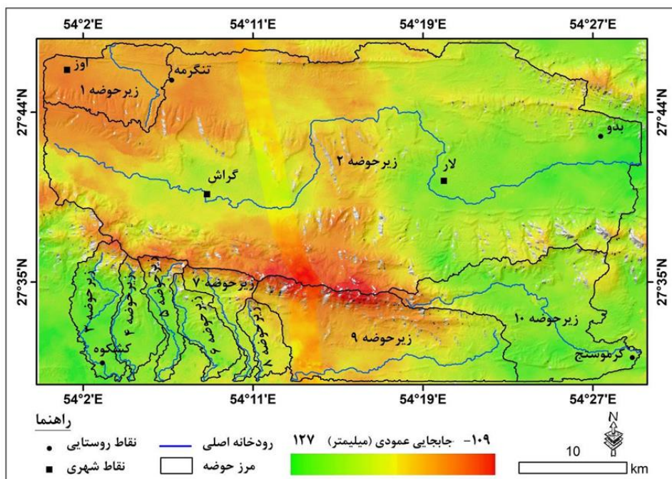
شکل ۵: نقشه میزان جابجایی عمودی منطقه از تاریخ (۲۰۲۰/۰۱/۱۲) تا (۲۰۲۲/۰۱/۰۱)
