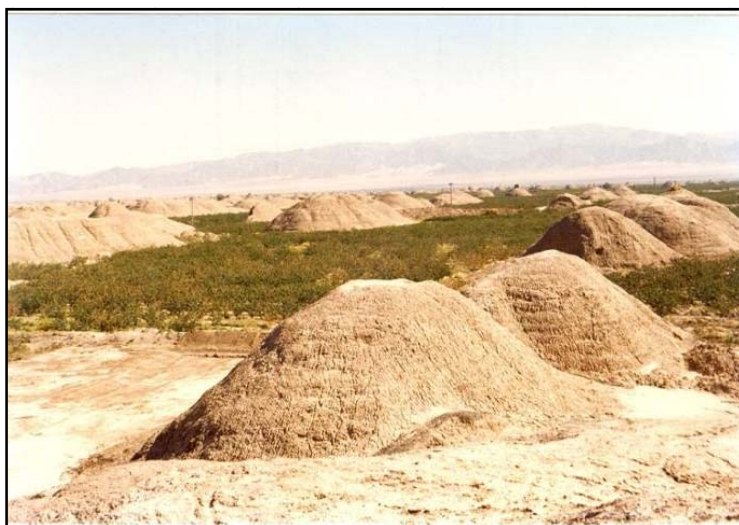
شکل ۵. تصویری از یاردانگ‌های شمال دشت رفسنجان که در آن کریدور بین یاردانگ‌ها پسته‌کاری شده است.
