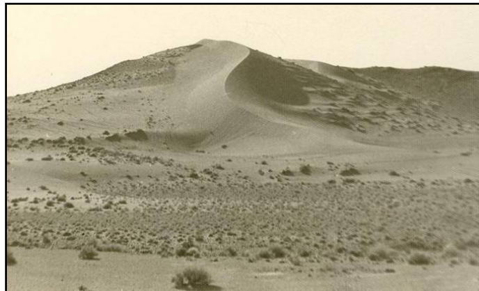
شکل ۹. تصویری از یک تلماسه‌ی سیف در شمال شرق دشت رفسنجان
