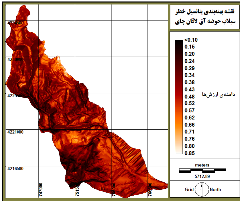
شکل ۱۱: نقشه پهنه‌بندی خطر سیلاب حوضه‌ی آق لاقان چای
